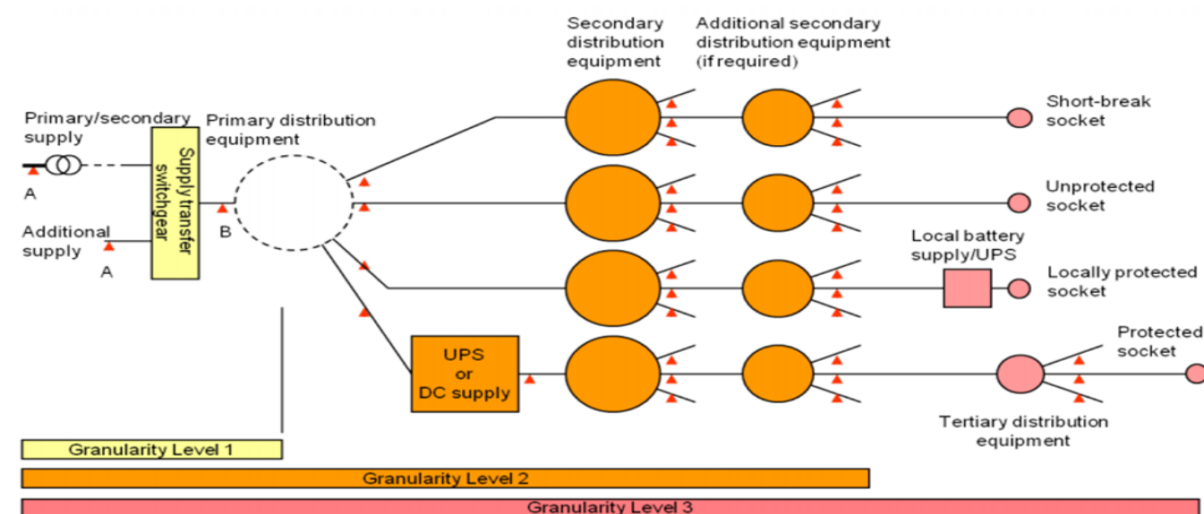
Ilustración 4 Criterios de diseño según disponibilidad
