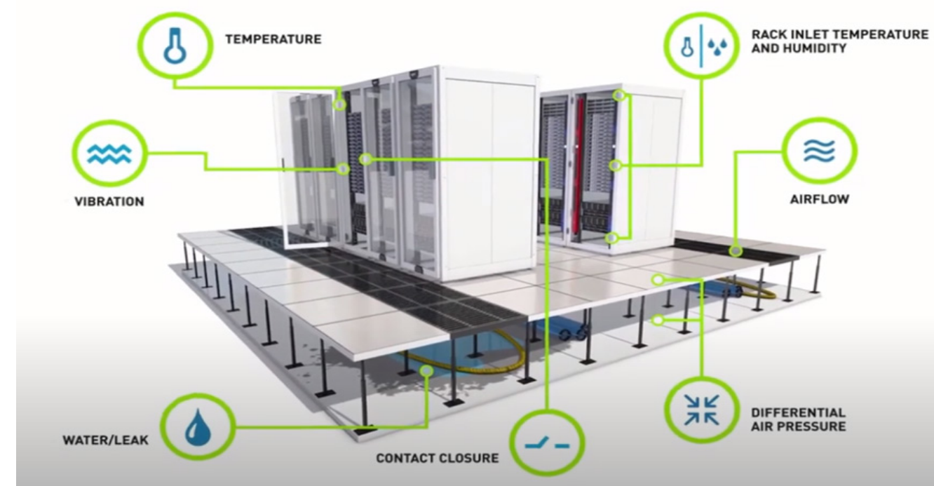
Esquema de concepto ambientales
