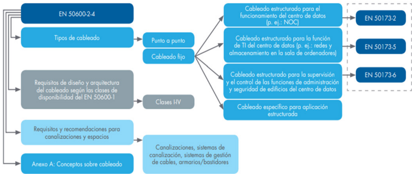
Cuadro resumen cableado
