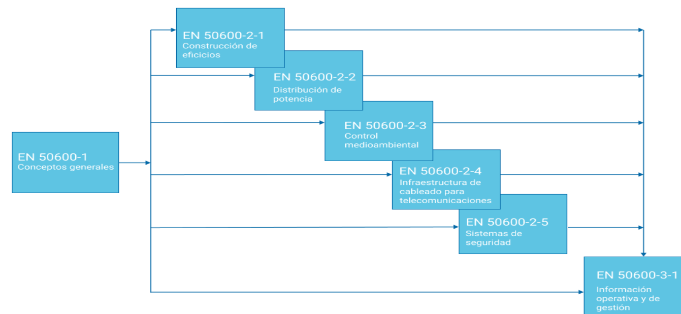
Estructura del EN 50600
